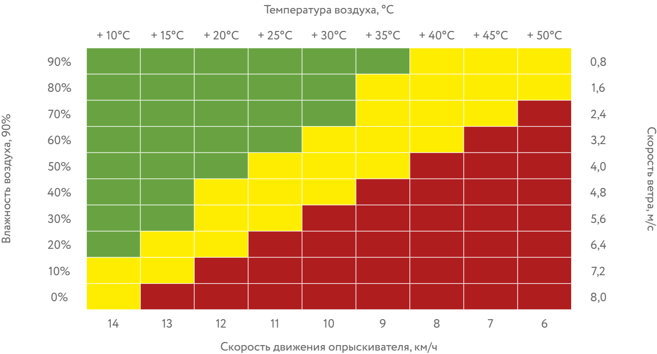
Корреляция скорости ветра, температуры, влажности воздуха в течении дня планирования опрыскивания
