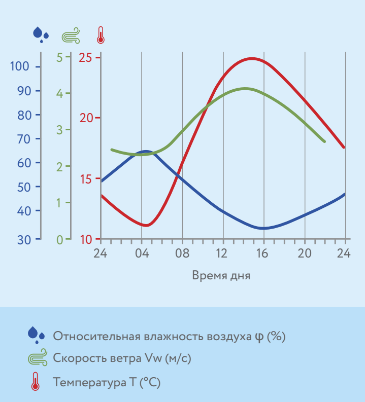
Корреляция скорости ветра, температуры, влажности воздуха в течении дня планирования опрыскивания
